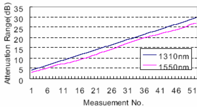
Variable Attenuator(Air-Gap:UPC-APC)
